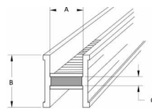
Staallood H 12 x 4,5 lengte 2 meter (STH8x45M2)
